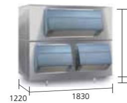
B 3200 Накопитель льда 1500 Кг
