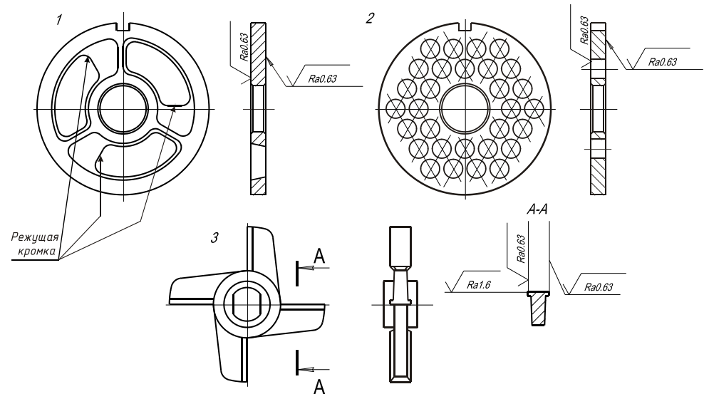
1 - Нож подрезной; 2 - Решётка; 3 - Нож двусторонний Рисунок 8 – Заточка ножей и решётки
